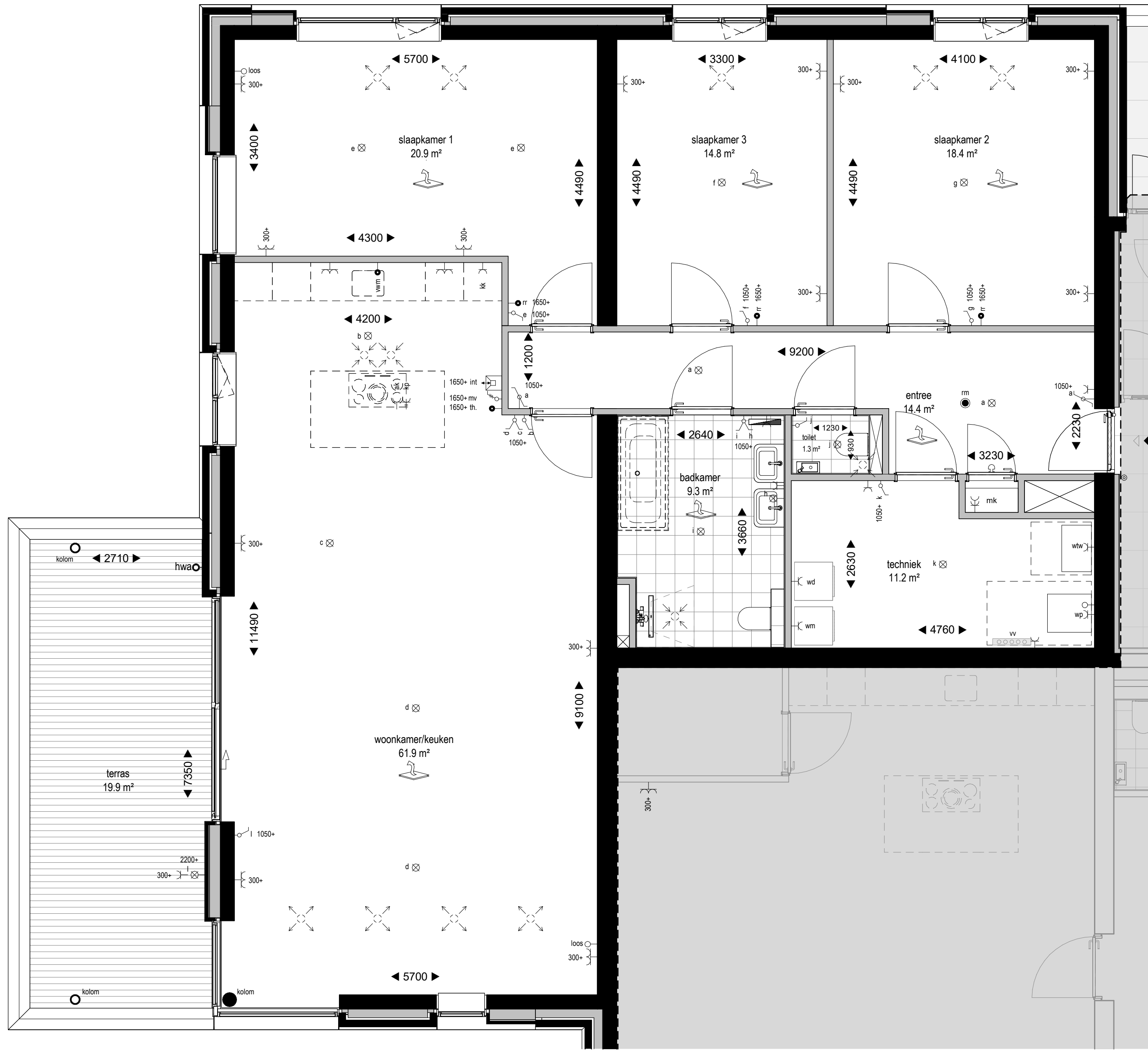
Begane grond - bouwnummer 64 1 : 50
