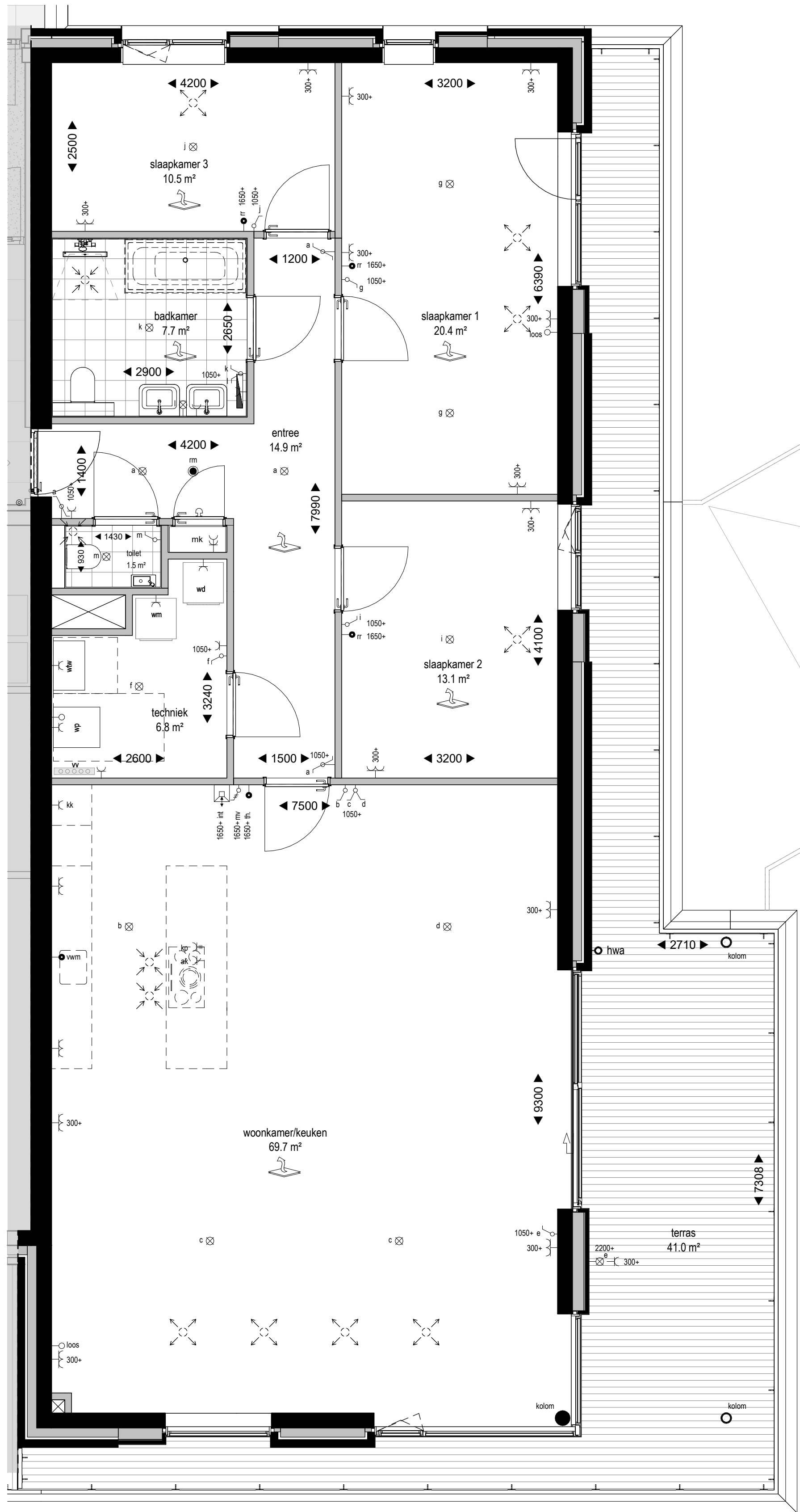
Begane grond - bouwnummer 66 1 : 50
