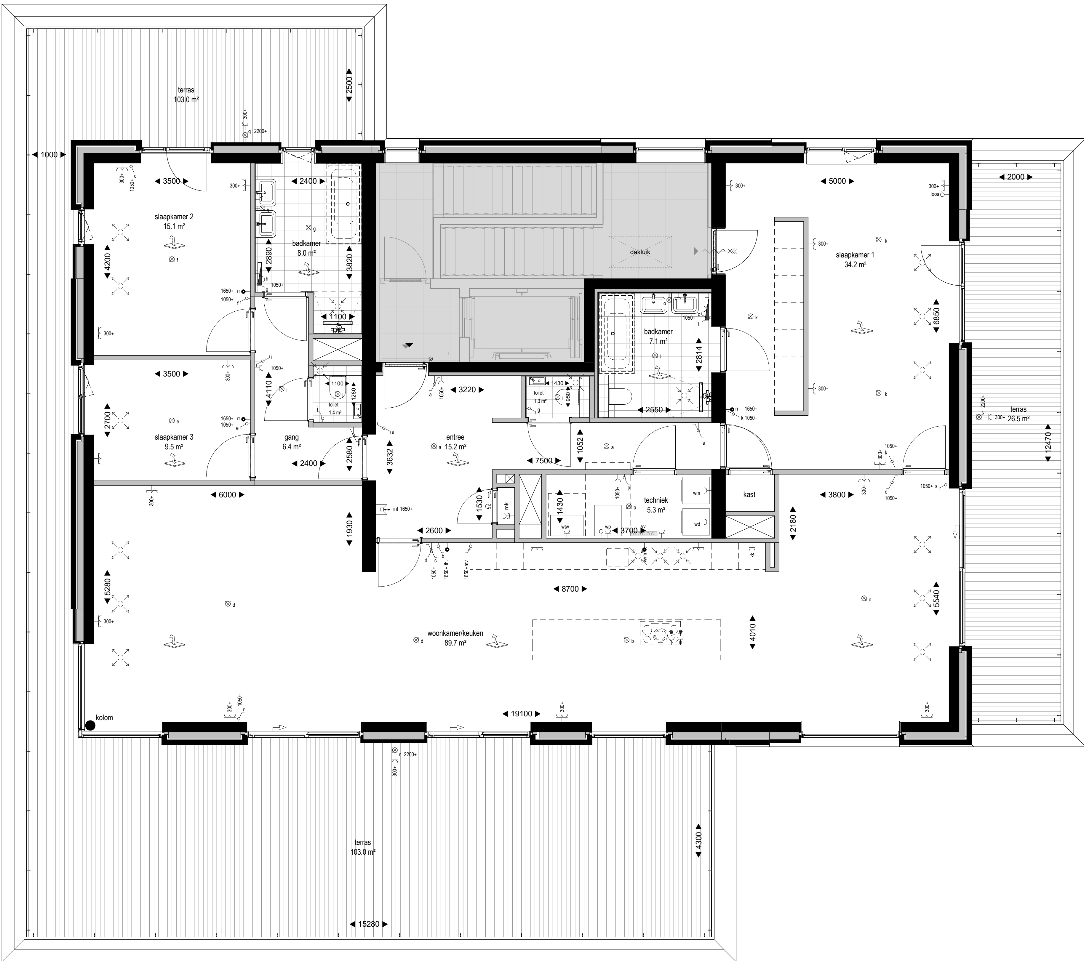
Derde verdieping - bouwnummer 72 1 : 50
