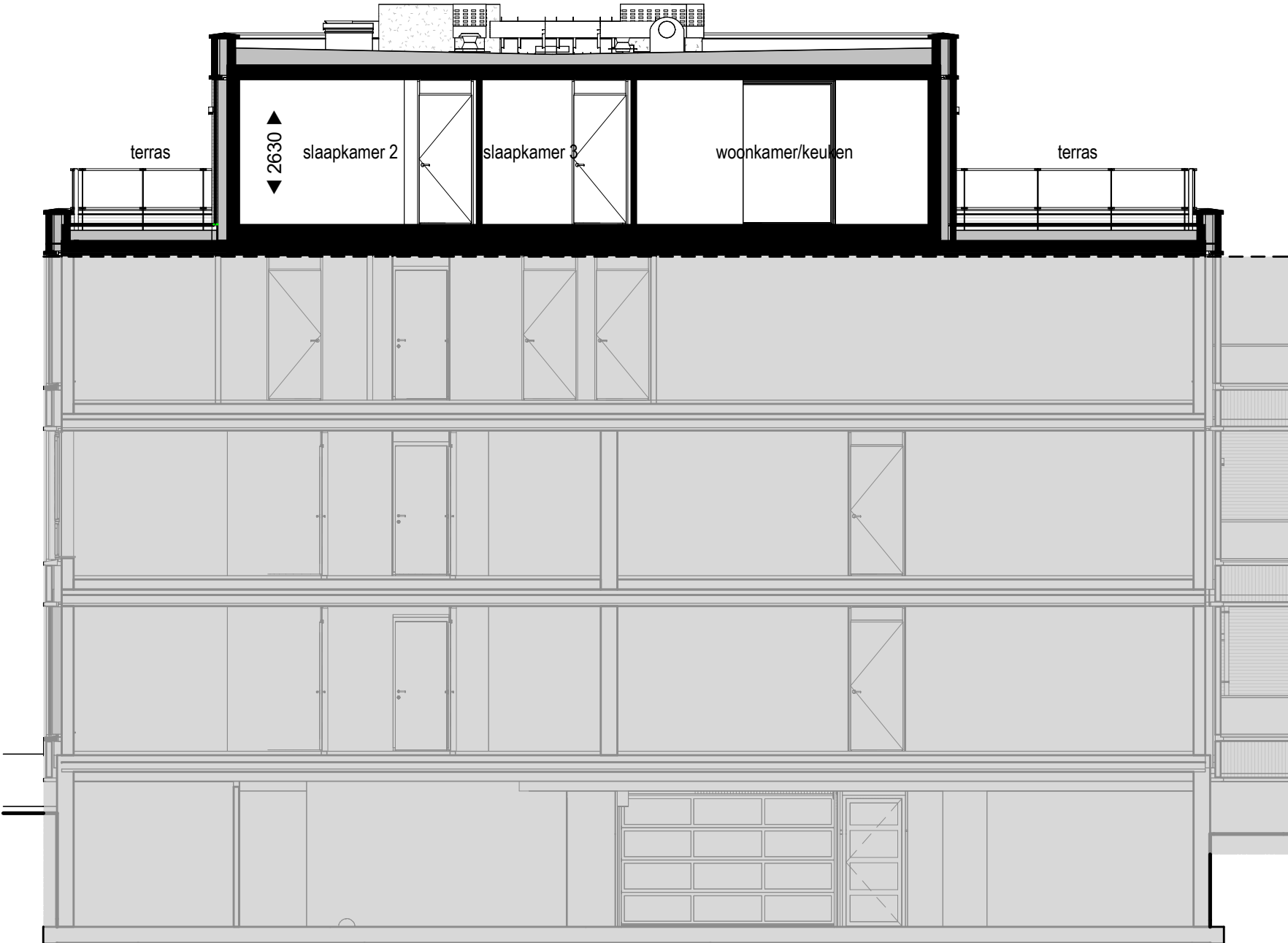
Doorsnede - bouwnummer 72 1 : 100
